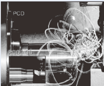
チップブレーカなしでの 切りくず排出
